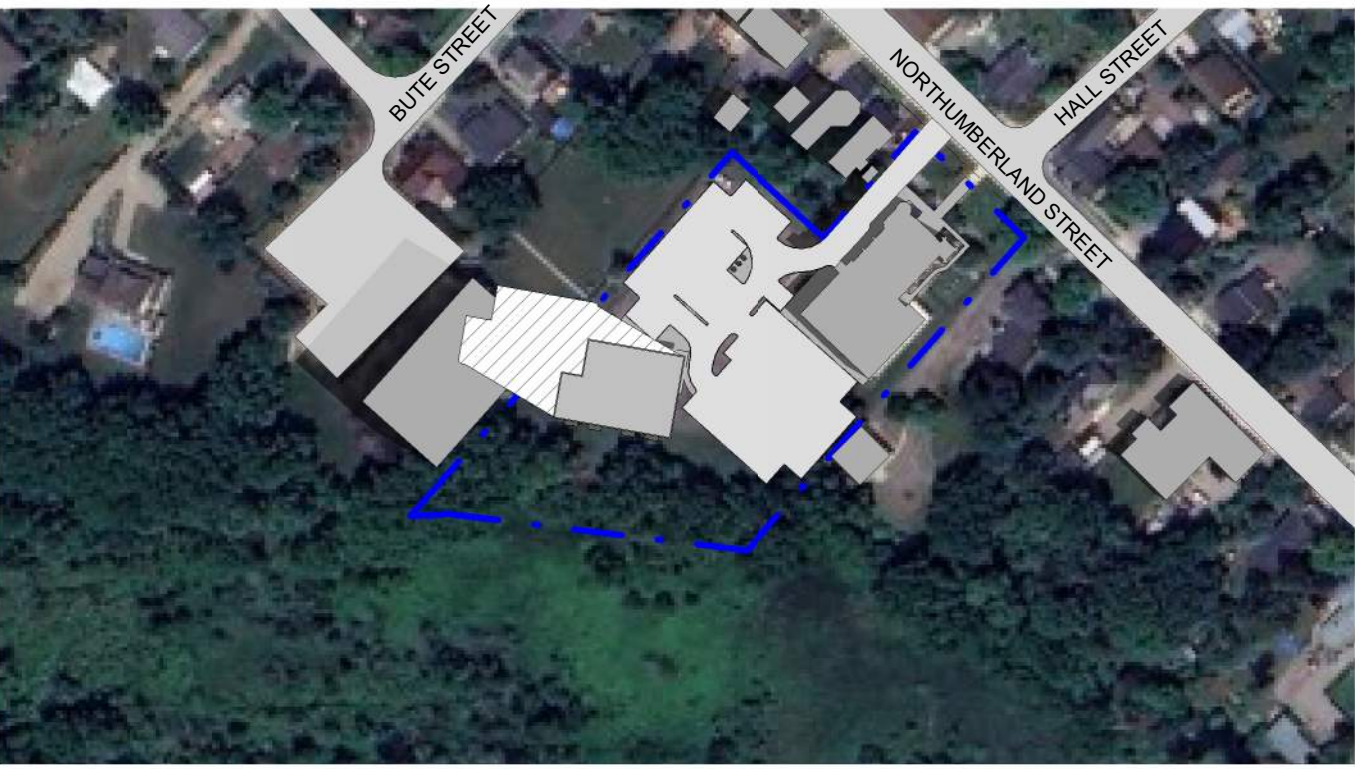
2 Shadow Study September 21 9am 1 : 2000
