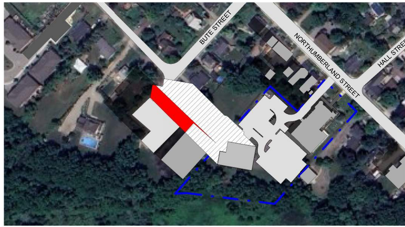
1 Shadow Study December 21 9am 1 : 2000
